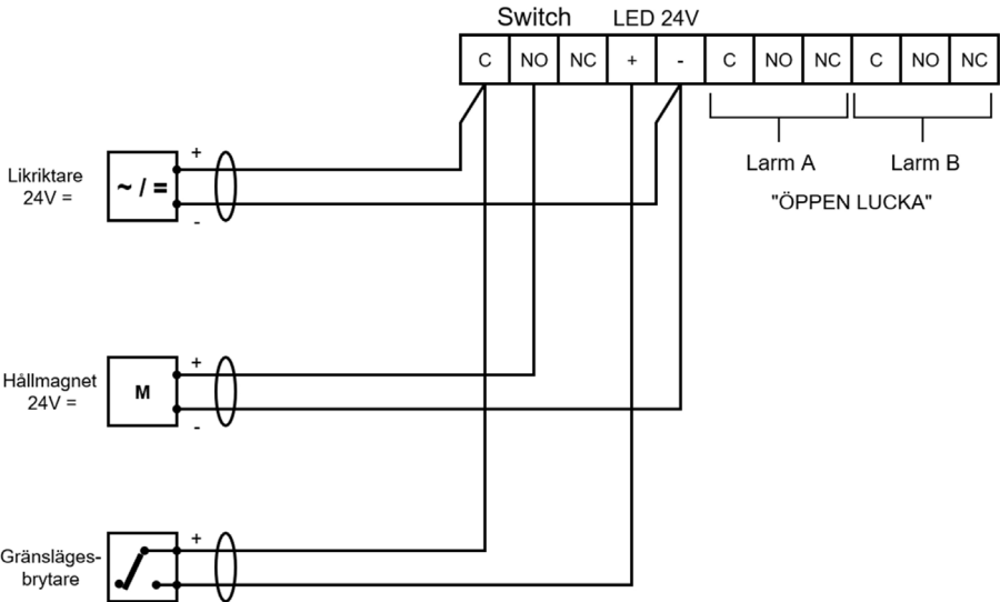
INKOPPLINGSEXEMPEL NB-3-REL
